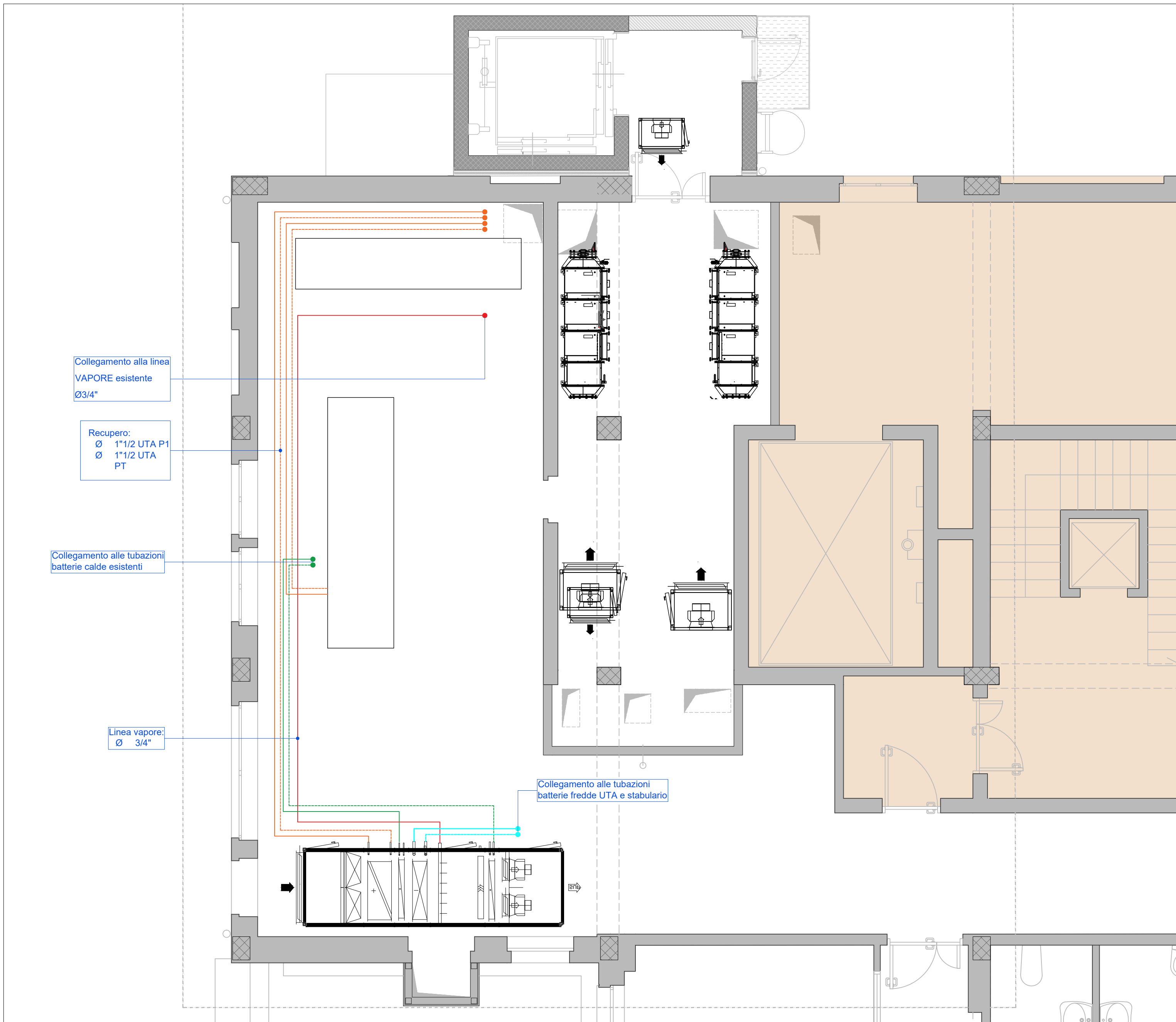
Pianta piano Secondo scala 1:50
